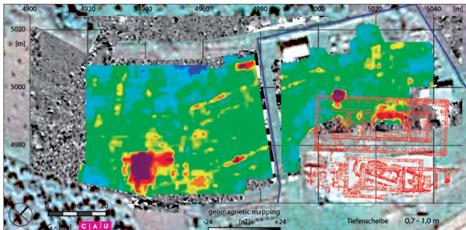
2 Καλαπόδι, αποτελέσματα της γεωμαγνητικής και γεωηλεκτρικής διασκόπησης στην περιοχή δυτικά των ναών | Kalapodi, Ergebnisse der geomagnetischen und geoelektrischen Prospektion im Areal westlich der Tempel
