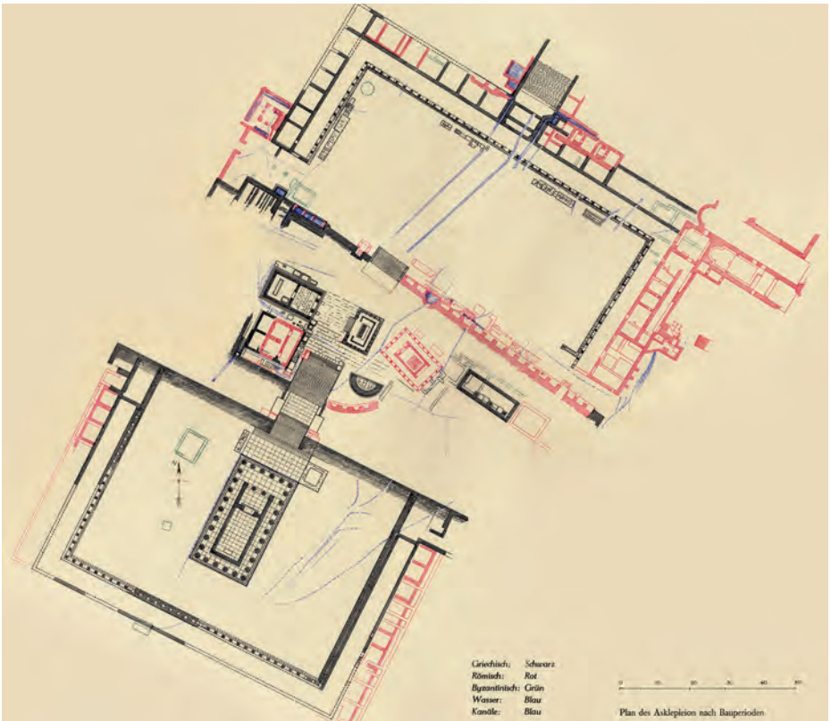
4 Κως, σχέδιο του ιερού του Ασκληπιού κατά Schazmann, επικαλυμμένο με τα αποτελέσματα της φωτογραμμετρικής αποτύπωσης | Kos, Plan des Asklepiosheiligtums nach Schazmann, überlagert mit den Ergebnissen der fotogrammetrischen Auswertung
